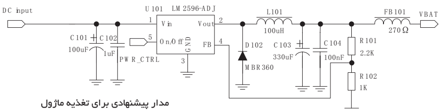
مدار پیشنهادی برای تغذیه ماژول
